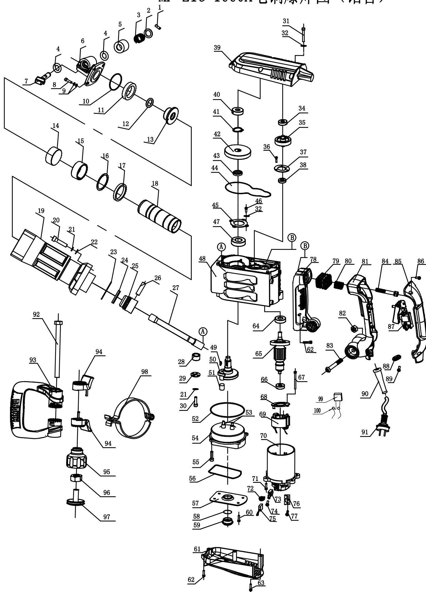
MP-Z1G-1660A电镐爆炸图 (铭普)
